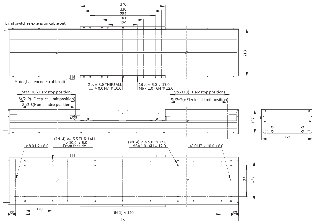
■ DGL200-AKM50-B4 尺寸图
