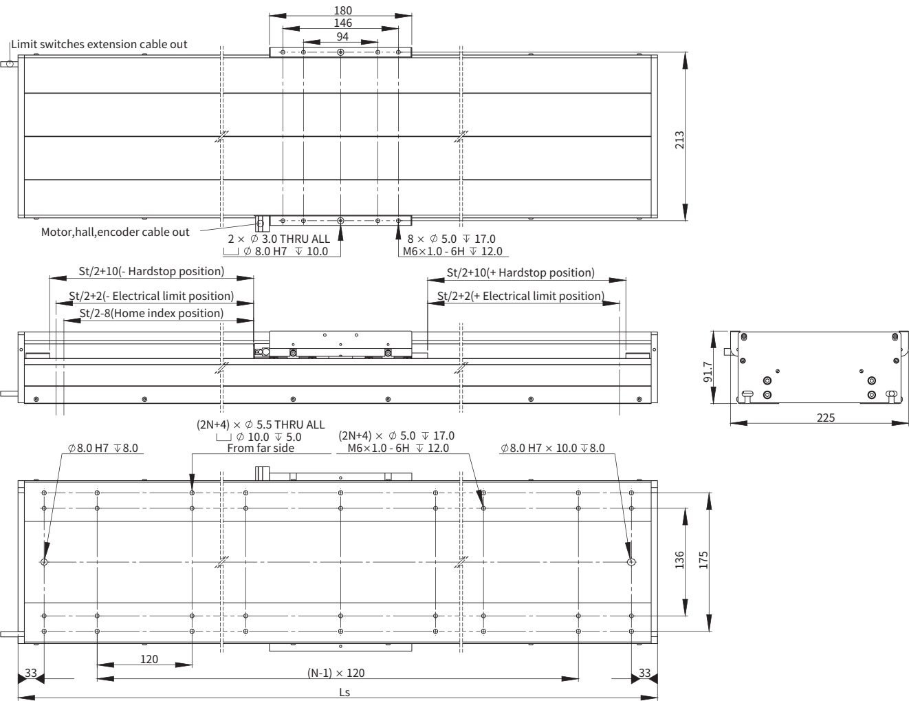
DGL200-AJM80-B2 尺寸图
