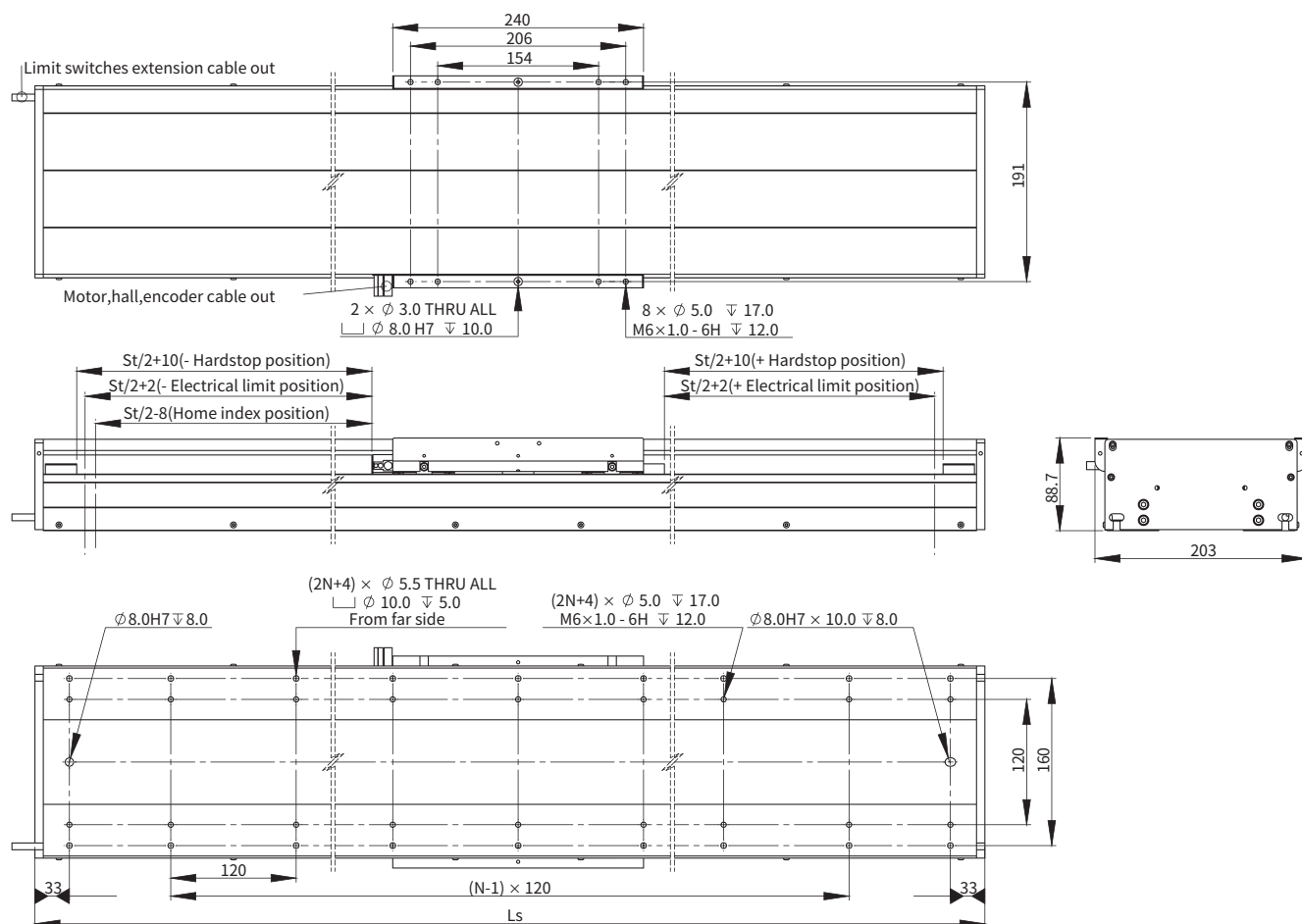
■ DGL180-AJM50-B4 尺寸图
