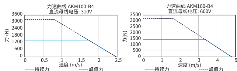
■ 力-速度 曲线
