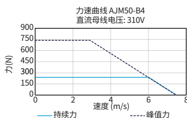
■ 力-速度 曲线
