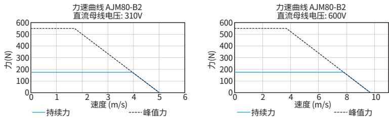
■ 力-速度 曲线
