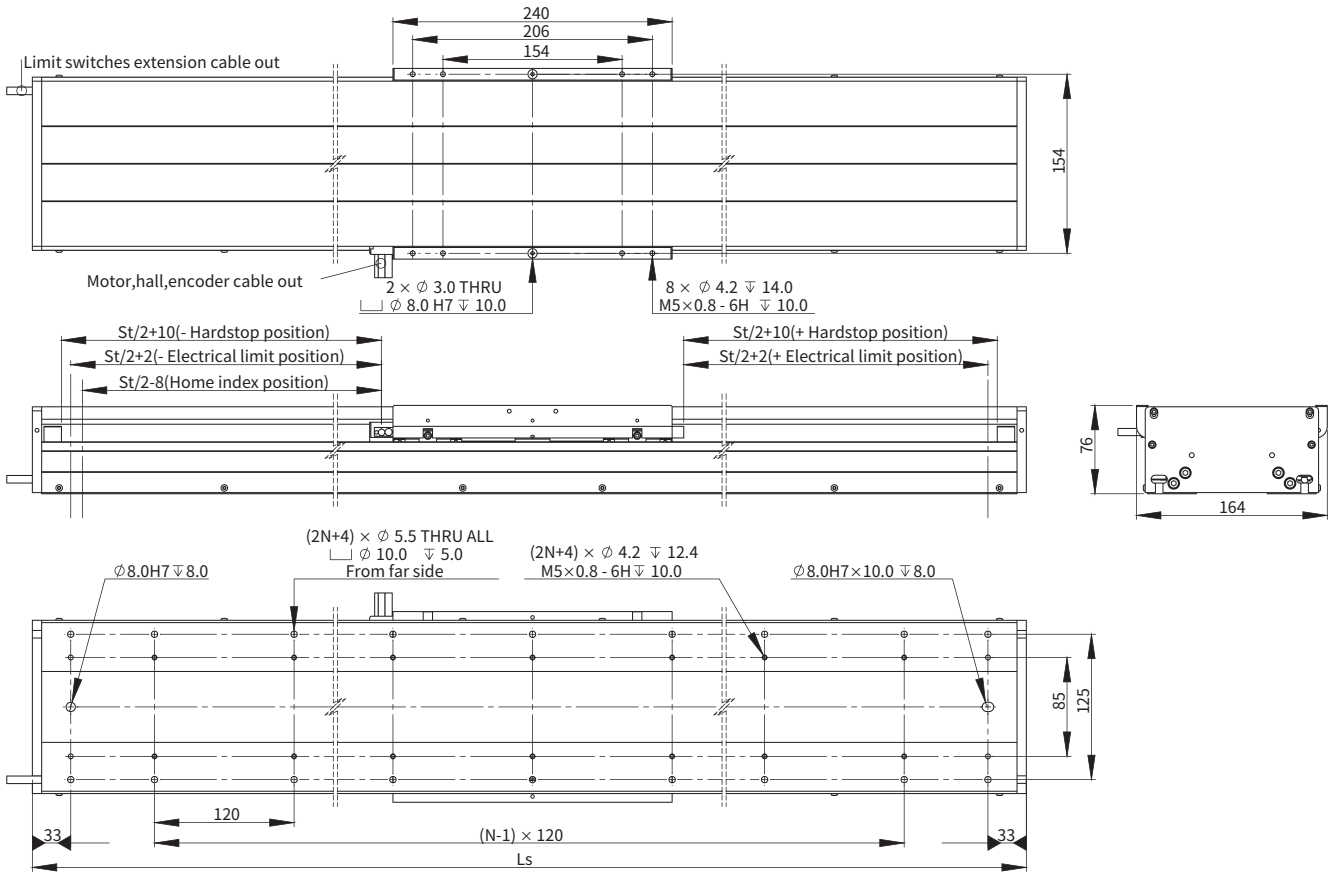
DGL150-AJM30-B4 尺寸图
