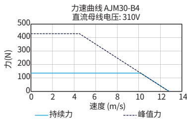
■ 力-速度 曲线
