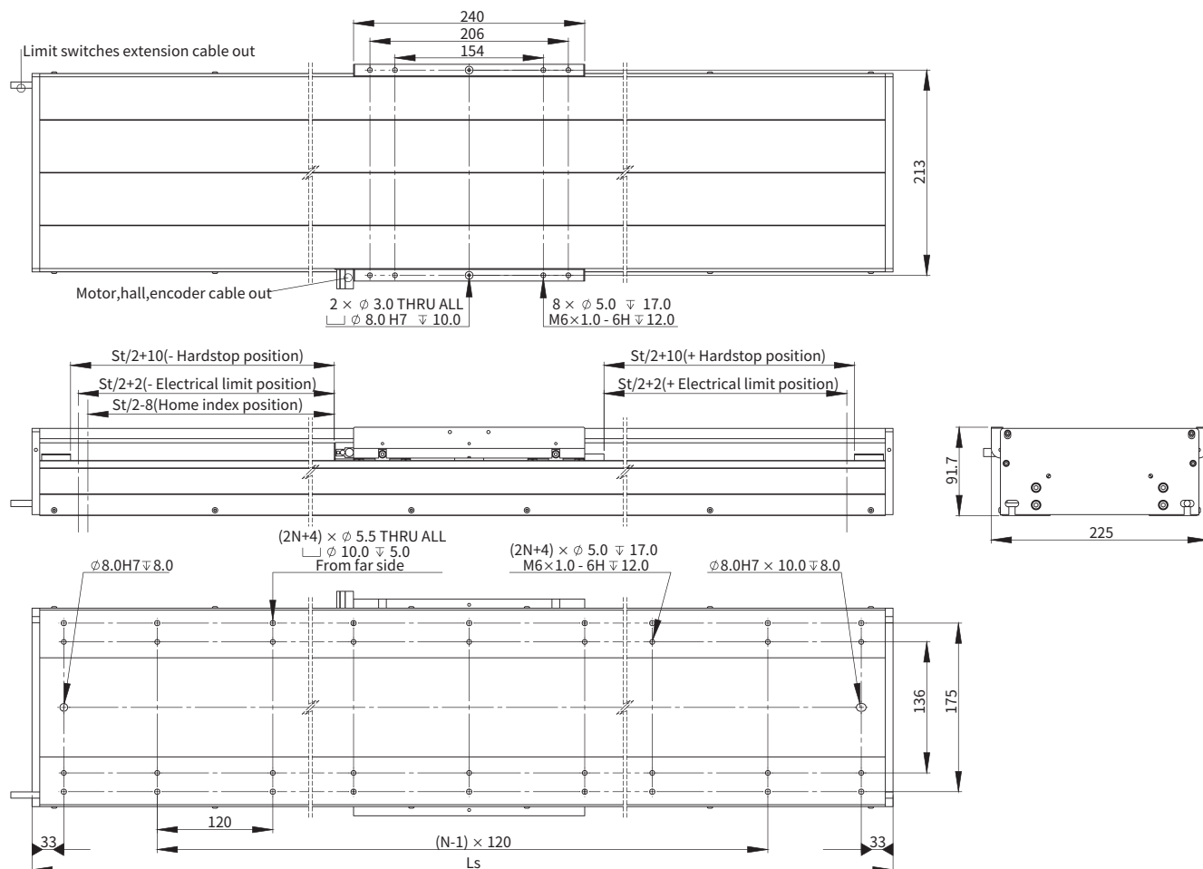
■ DGL200-AJM80-B4 尺寸图
