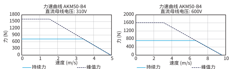
■ 力-速度 曲线
