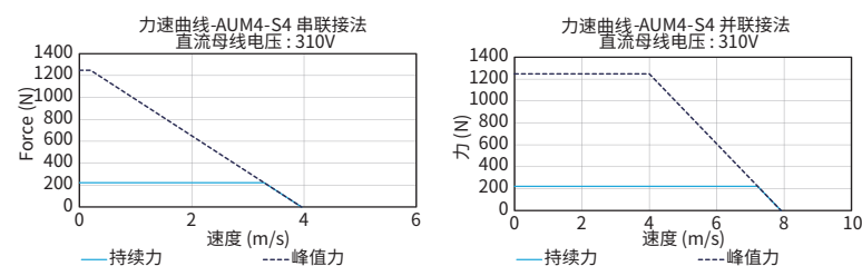
■ 力-速度 曲线
