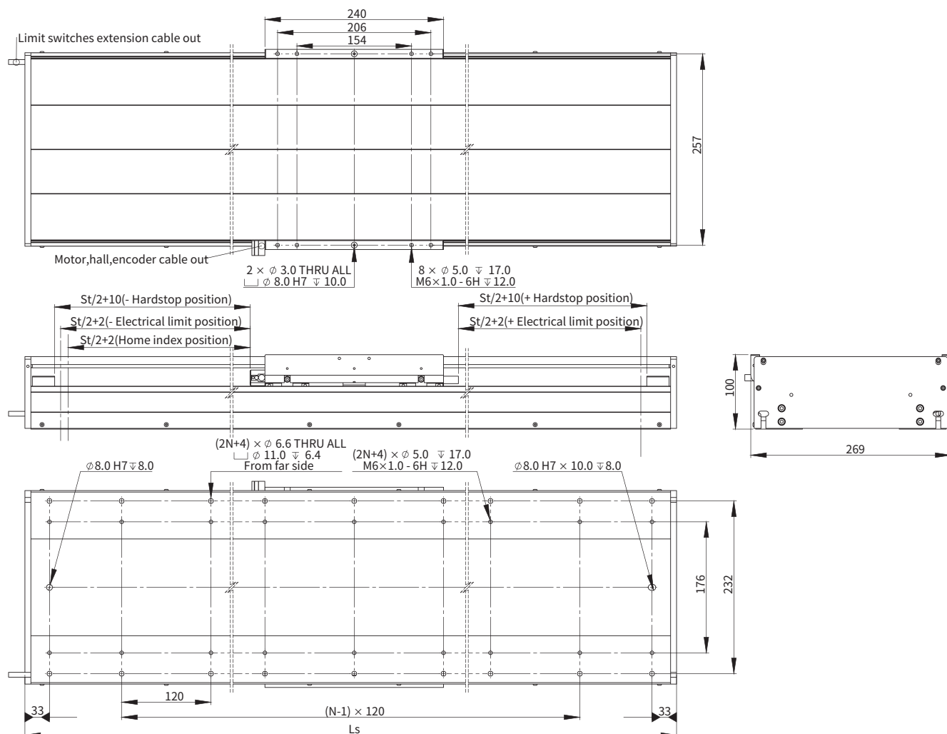
■ DGL260-AJM100-B4 尺寸图
