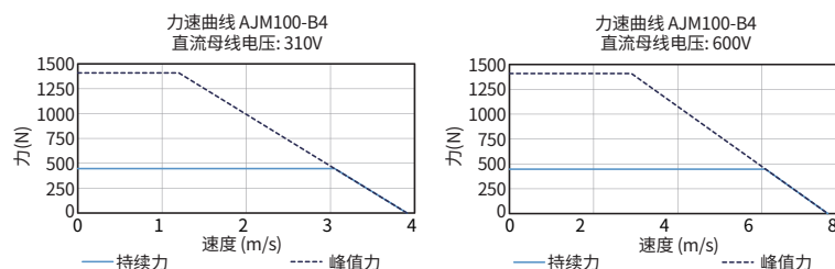
■ 力-速度 曲线
